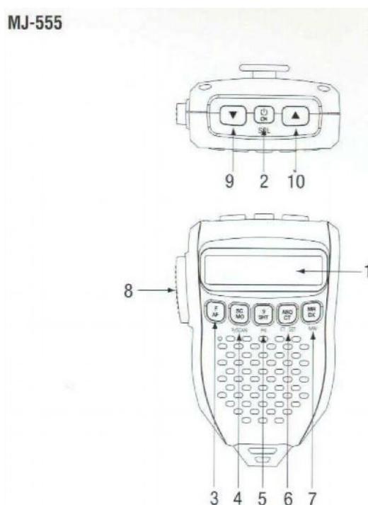
Рис. 3. Тангента радиостанции MegaJet MJ-555
