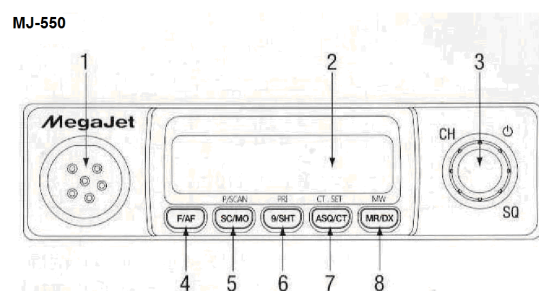
Рис. 1. Органы управления радиостанции MegaJet MJ-550
